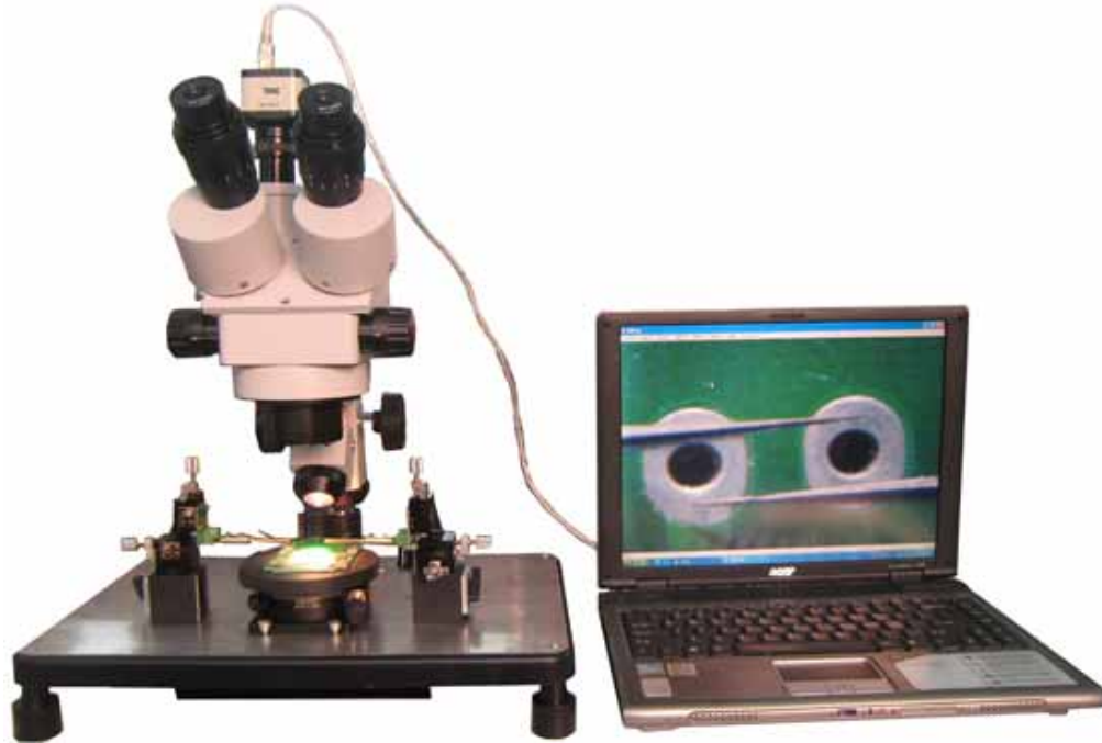
显微镜和 USB 接口 CCD 摄像头共存的监视方式
